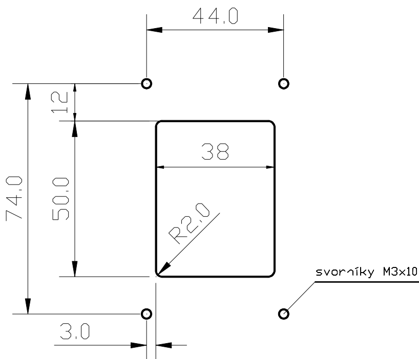
Výkres otvorů pro umístění MPS v ovladači
